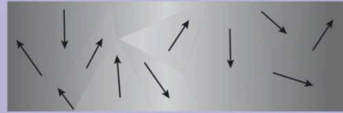
المناطق المغناطيسية
